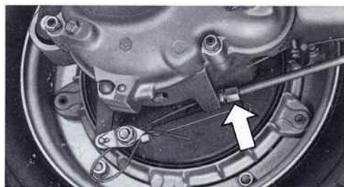
Fig. 16 - Registrazione freni
