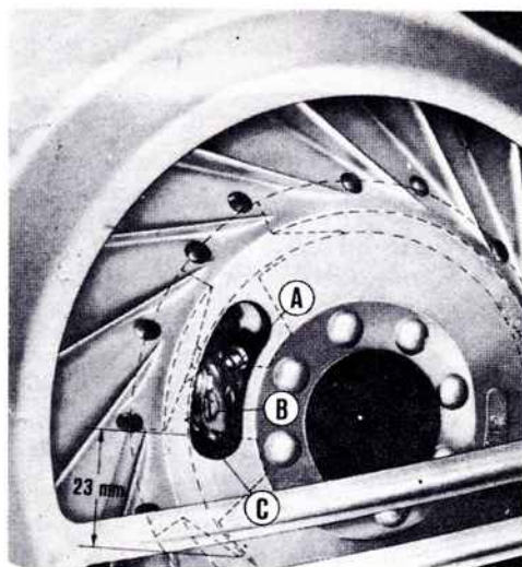
Fig. 4 - Operazioni per il controllo della fasatura (P125X - P150X).
