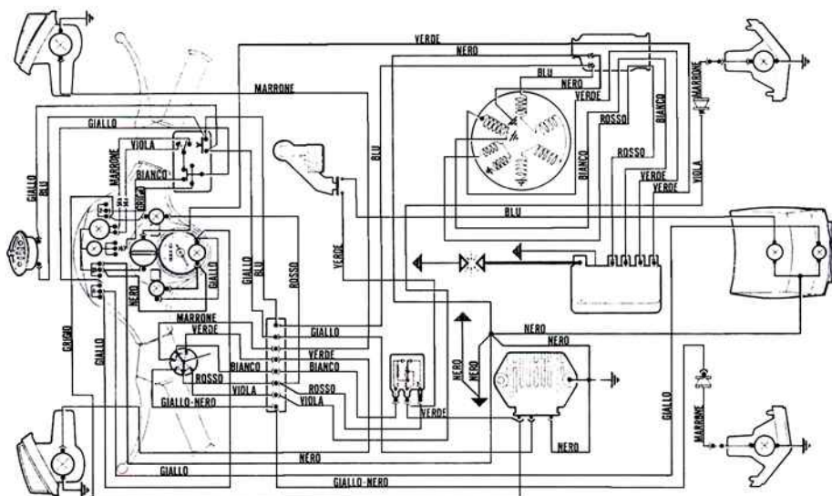
Fig. 2 - Schema impianto elettrico (P200E)
