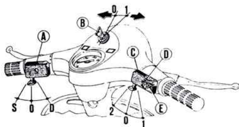
Fig. 3 - Posizioni dei commutatori.
